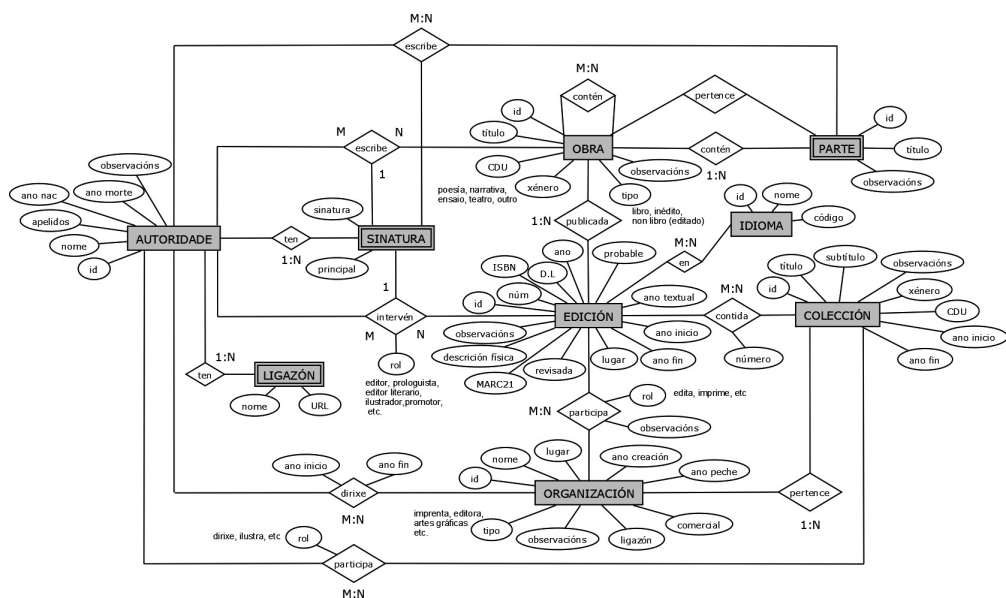
Fig. 1. Diagrama Entidade-Relación.
